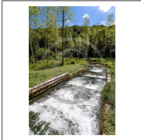
Isère (38), commune de Saint-Blaise-du-Buis, Le Rivier, Espace naturel sensible de l'Isère, étang de Cote Manin, passe à poissons construite pour assurer la continuité écologique de la rivière La Fure // Isère (38), Saint-Blaise-du-Buis, Le Rivier, sensitive natural area of the Isere, pond Cote Manin, fishway built to ensure the ecological continuity of the river Fure
